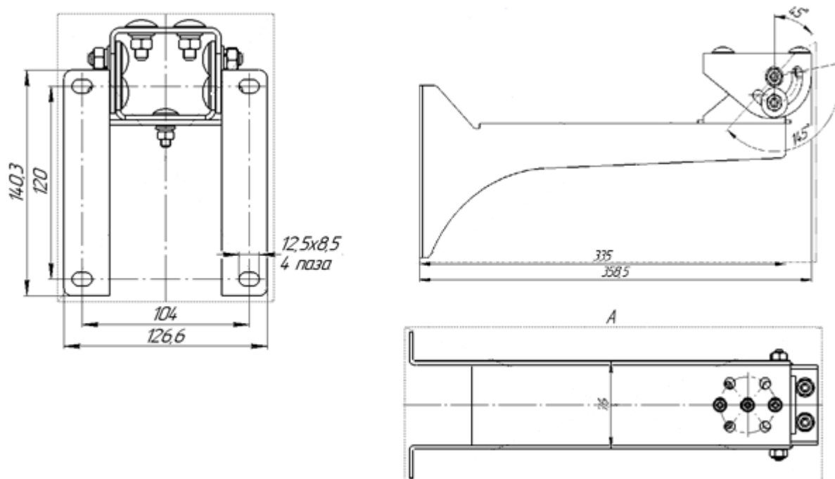
Рис. 1 – Габаритные размеры
