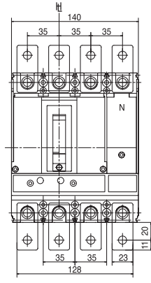
Детальный вид клемм
