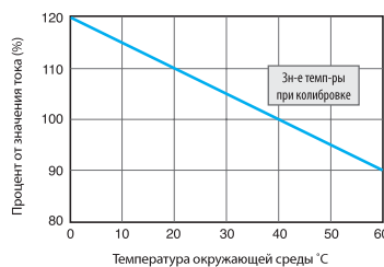
Компенсирование кривые окружающей среды
