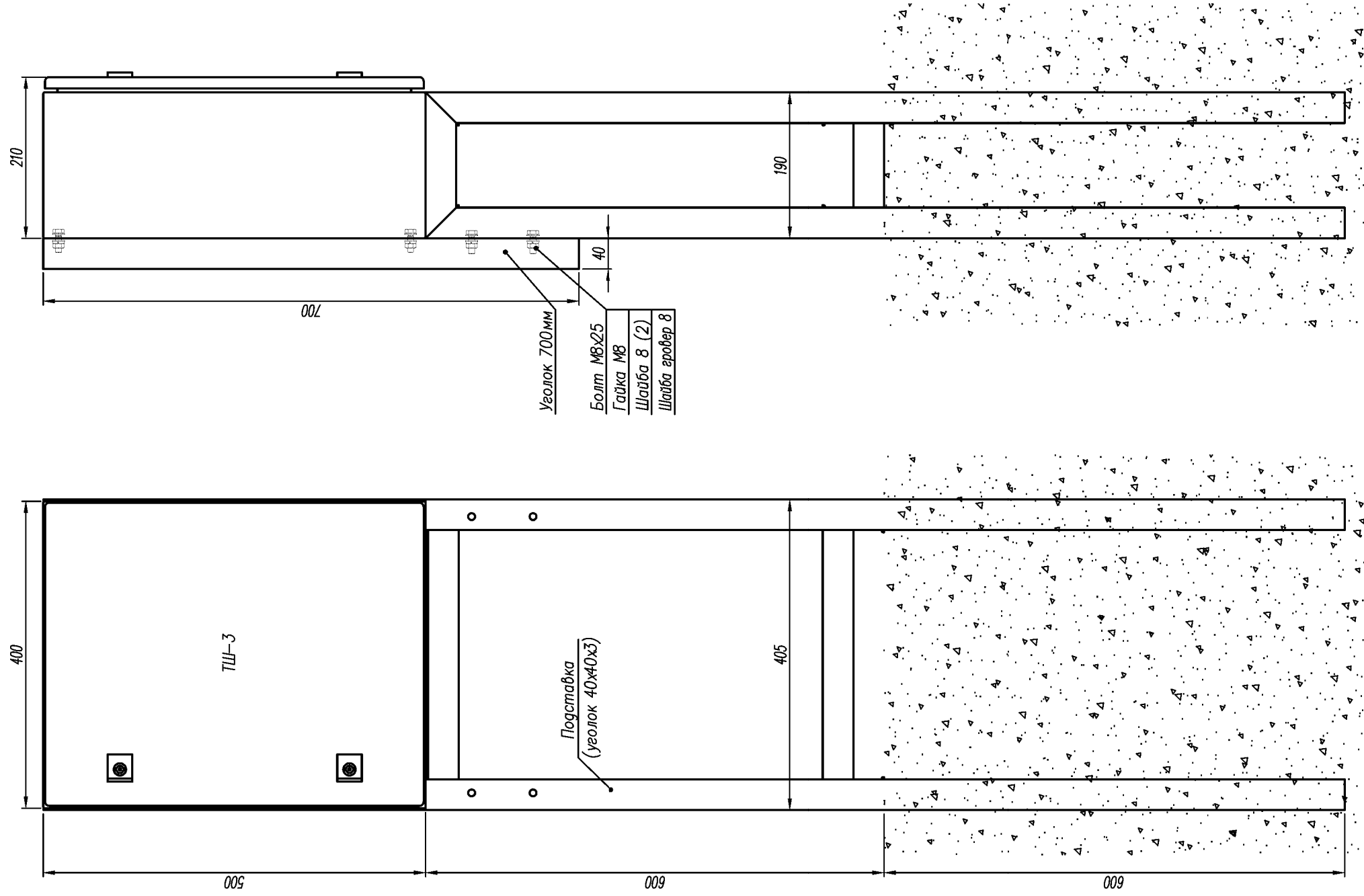
Рис.1 Габаритные и установочные размеры основания напольного ОНШ-3
