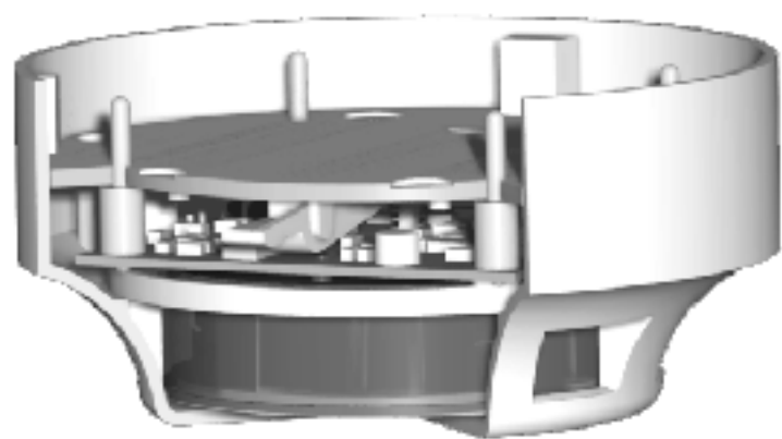
Рисунок 3 - Конструкция извещателя
