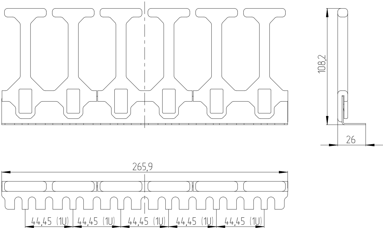
60A-18-06-16-09BL Вертикальный организатор Zero-U, 6U, с пластиковыми пальцами
