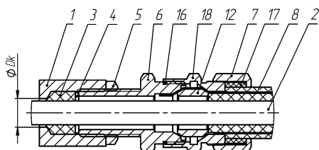
ж) монтаж бронированным кабелем в кабельном вводе KB5Y
