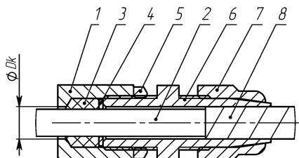
а) монтаж бронированным кабелем в кабельном вводе KB512
