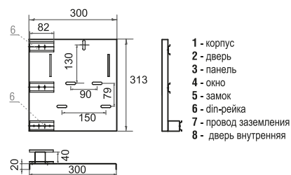
монтажная панель ЩУ 3/1-0
