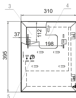
ЩУ 3/1-1 с оперативной панелью (дверцей)
