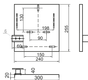
монтажная панель ЩУ 3/1-0
