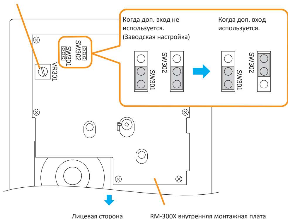
Регулирование громкости доп. входа
