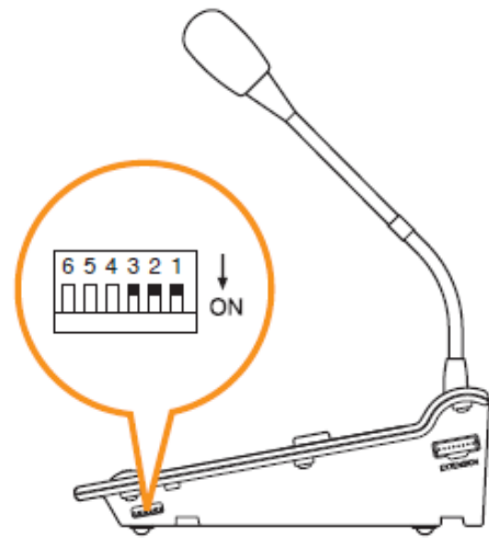
RM-300X сбоку
