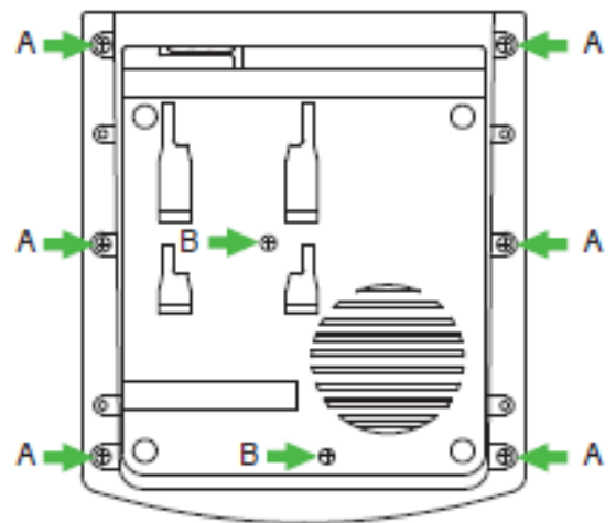
RM-300X снизу
