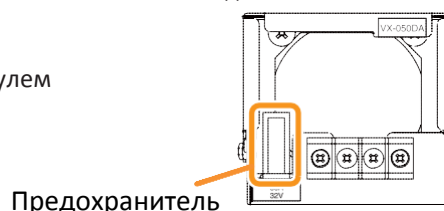
Задняя панель VX-015DA/030DA/050DA
