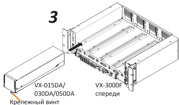
Крепежный винт
