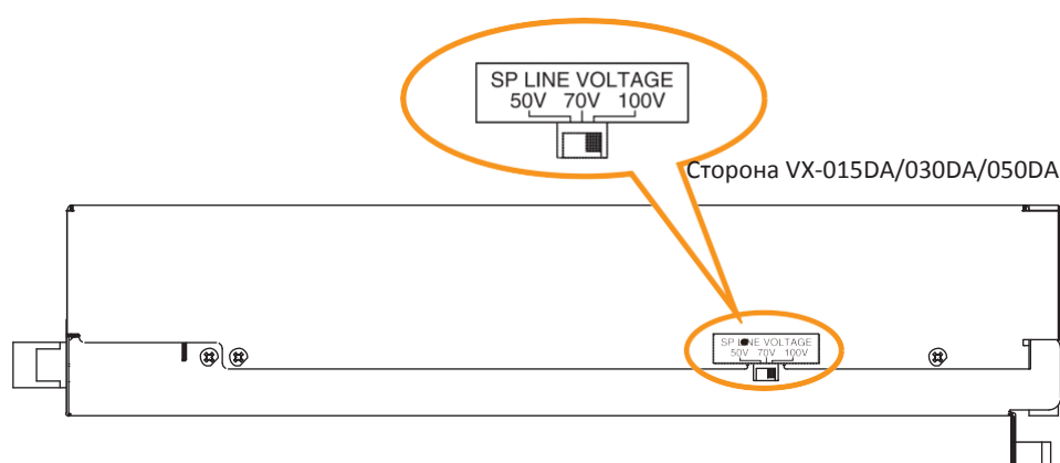
Селекторный переключатель выходного напряжения
