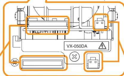
DA разъем линии управления
