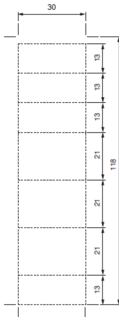
Этикетка с названием С Отрезаемый размер: 30 x 118 мм
