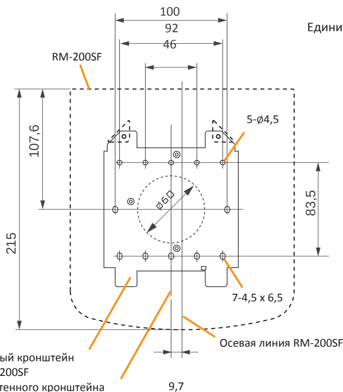
Настенный кронштейн (поставляется с RM-200SF)
