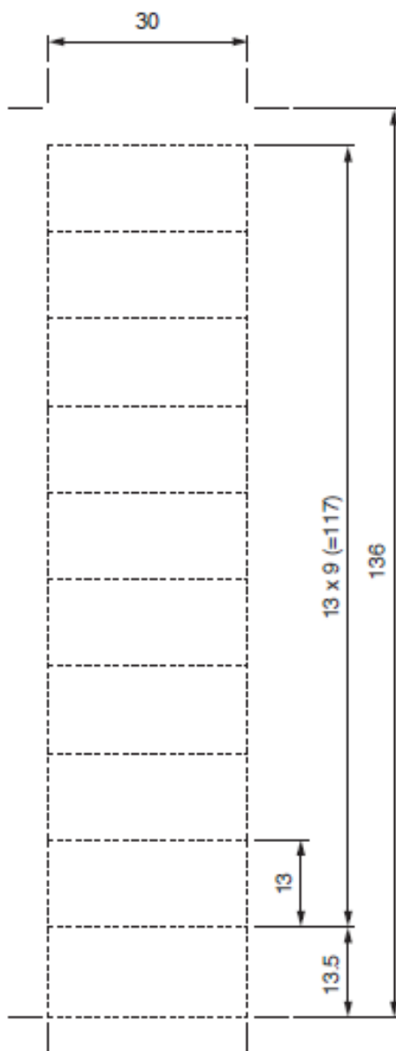
Этикетка с названием В Отрезаемый размер: 30 x 136 мм
