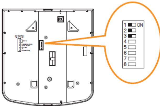
RM-200SF сзади
