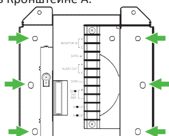
Настенный кронштейн (поставляется с RM-200SF)
