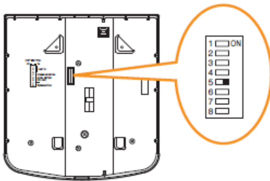
RM-200SF сзади
