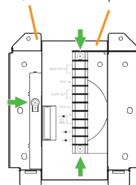
Настенный кронштейн (поставляется с RM-200SF)
