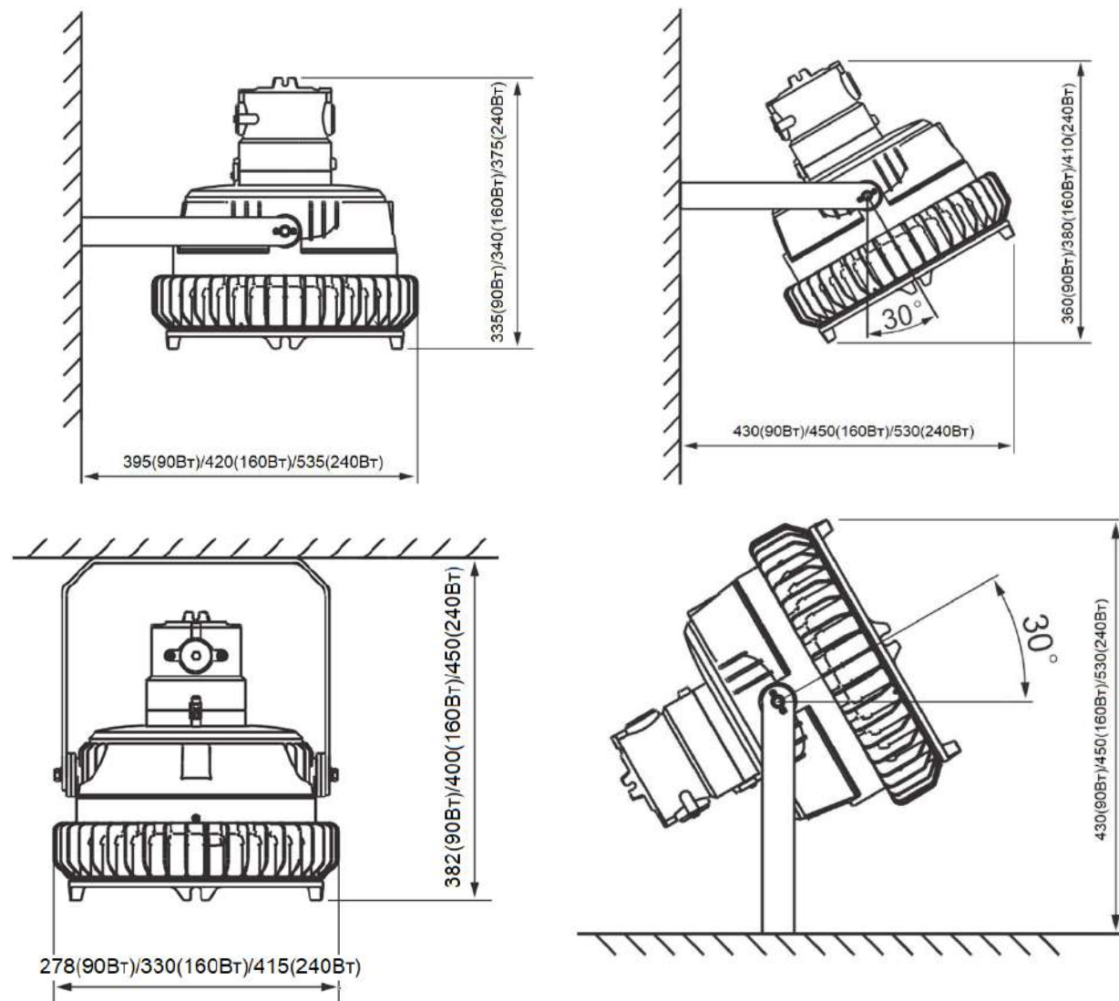
Рис. 1Б. Схема крепления светильников к опорной поверхности с помощью кронштейна.
