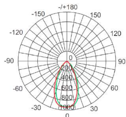
Светильник ЗЕНИТ МК 2.1-060 7200Лм. Светильник ЗЕНИТ МК 2.1-060 10450Лм. Примечание: Линзы 40° или 25° по запросу.
