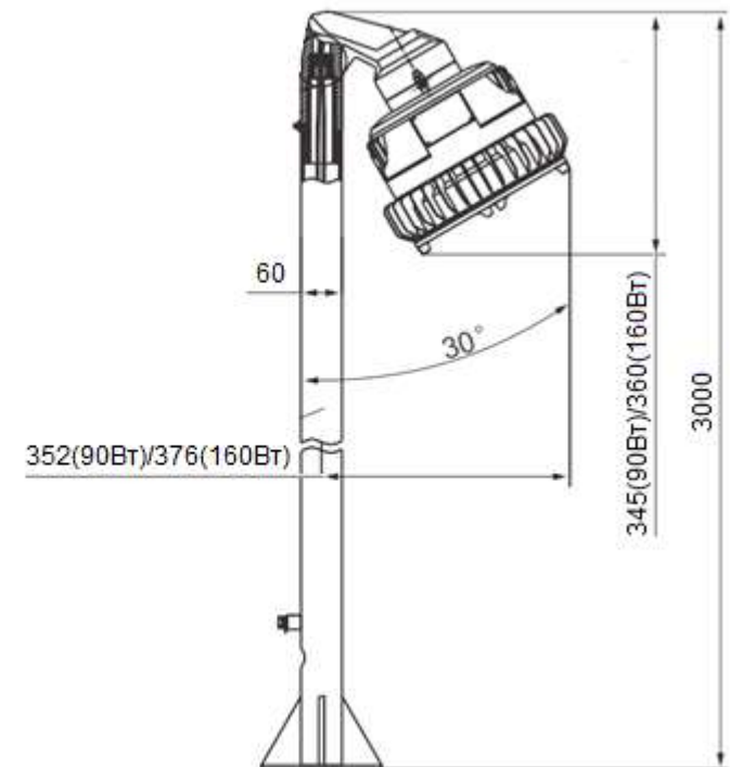
Рис. 4Б. Схема крепления светильника на световую опору.
