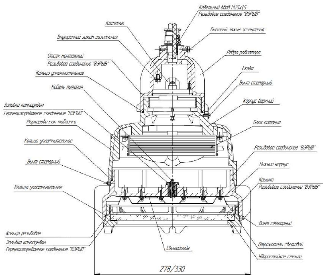
Рис. 1. Общий вид и детали конструкции взрывозащищенных светильников ЗЕНИТ МК 1.2-060, ЗЕНИТ МК 1.2-090, ЗЕНИТ МК 1.2-120, ЗЕНИТ МК 1.2-160
