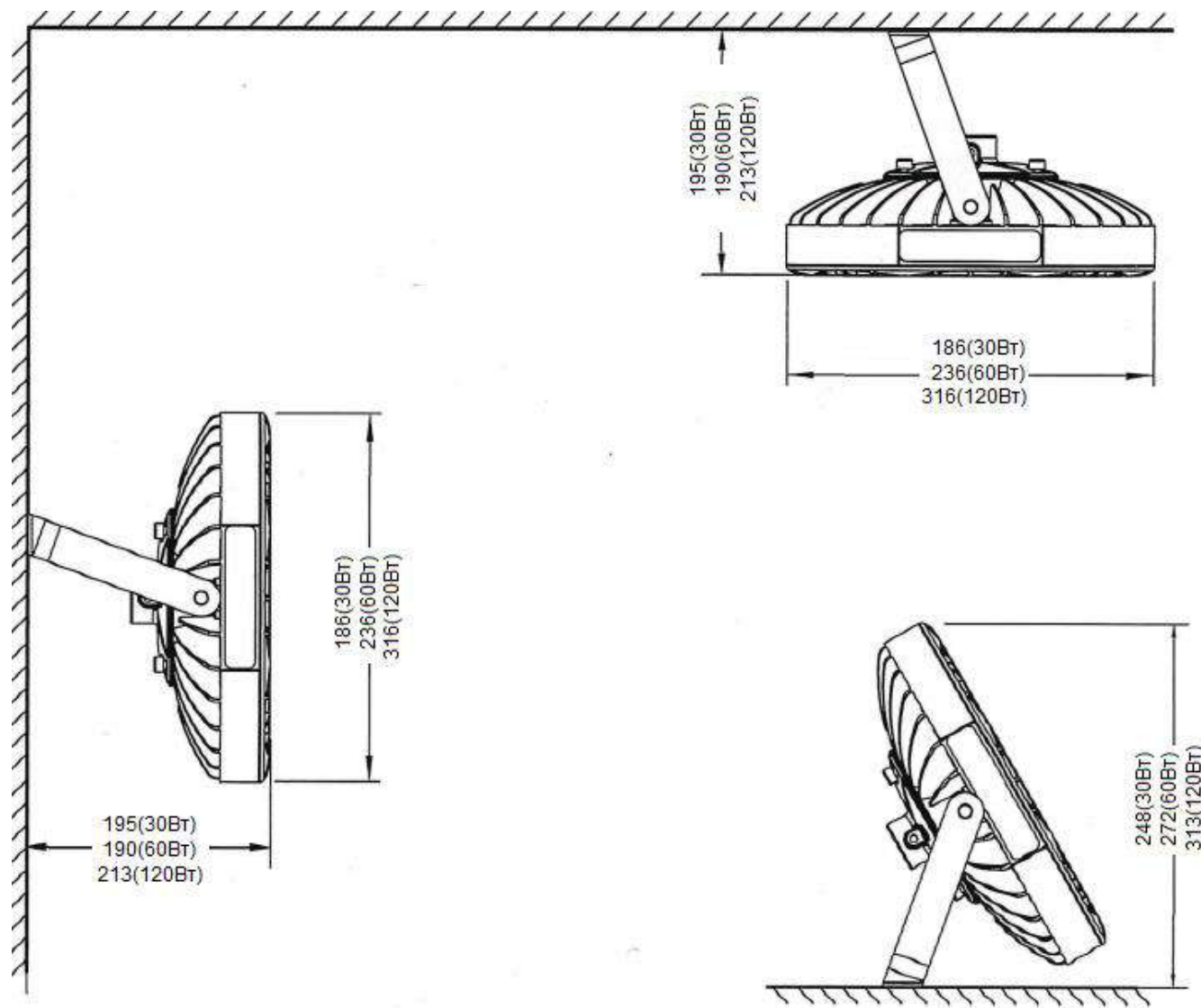
Рис. 1Б. Схема крепления светильников к опорной поверхности с помощью кронштейна.
