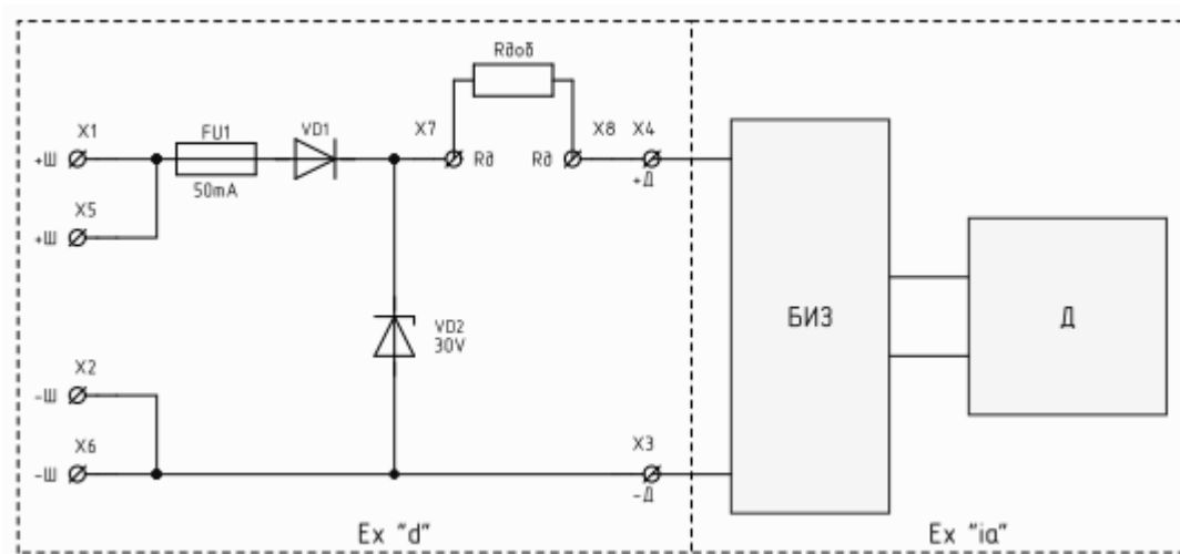
Рис.4 Извещатель ИП212 Трион МК. Схема принципиальная.
