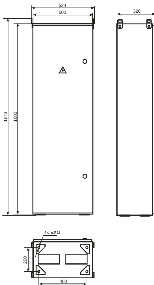
Рис.1. Внешний вид, габаритные и установочные размеры корпуса шкафа силового ШРС1-XX-5-Узола.
