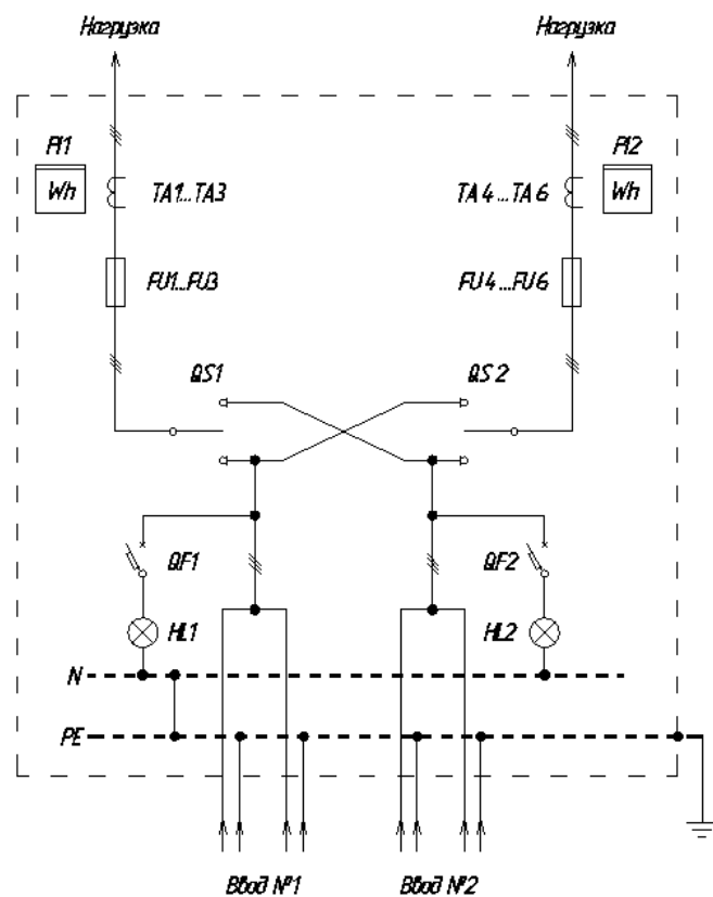
Рис.1 Схема электрическая принципиальная.
