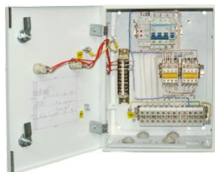
ЩР АВР 25А Узола
