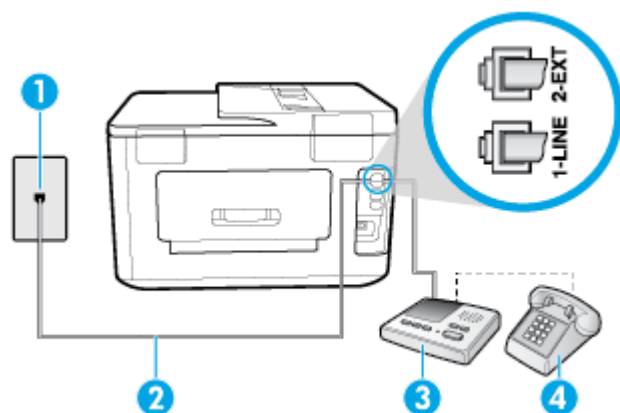
Рисунок 5-11 Вид принтера сзади
