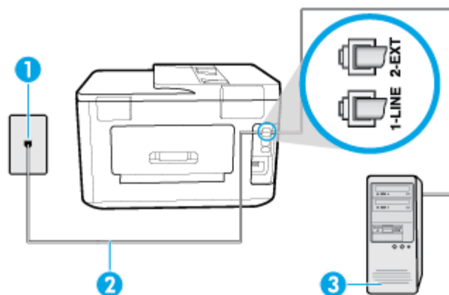
Рисунок 5-6 Вид принтера сзади
