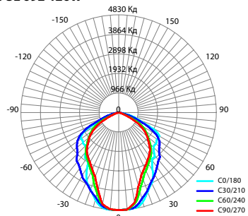
Кривая светораспределения светильника PSL 692-126W
