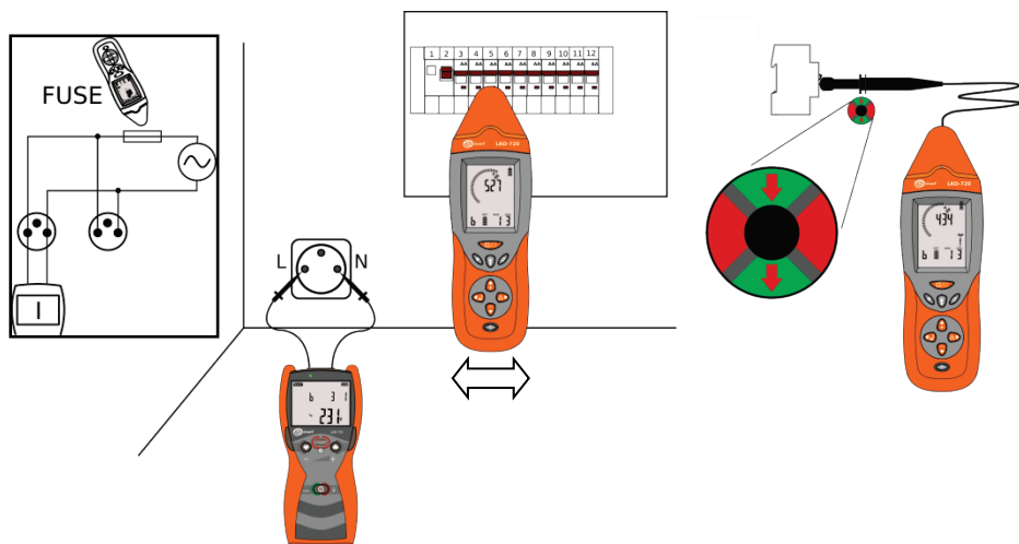
Рис. 27 Идентификация предохранителей в распределительном щитке.
