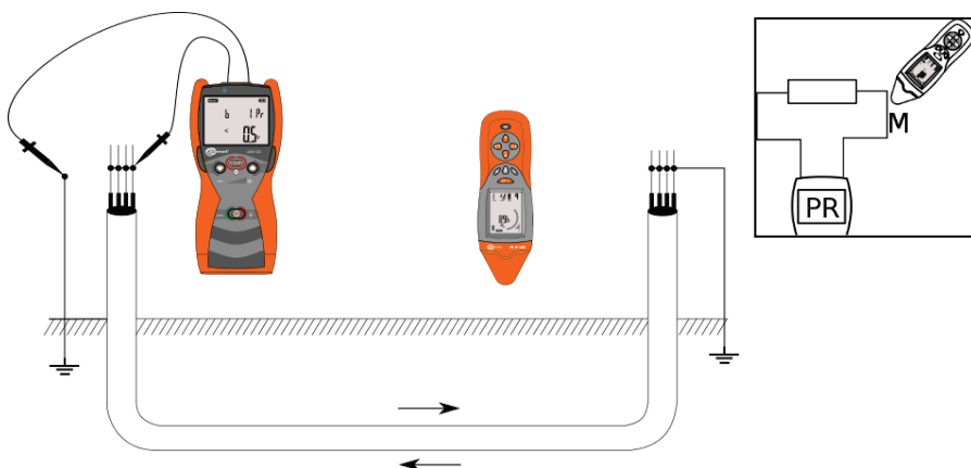
Рис. 28 Поиск кабеля с замкнутыми жилами в режиме «мощность»
