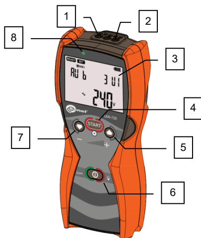
Рис. 1 Лицевая панель.
