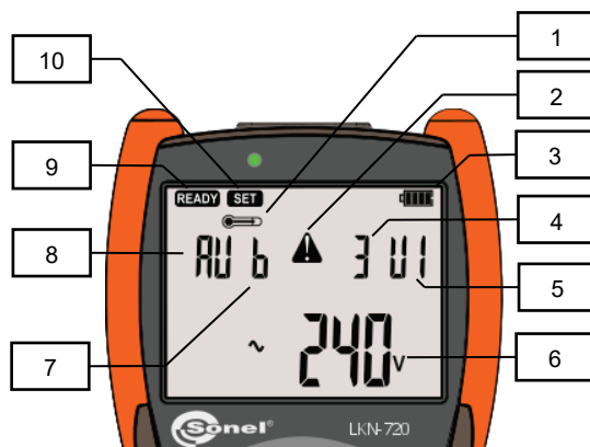
Рис. 2 Генератор - Дисплей.
