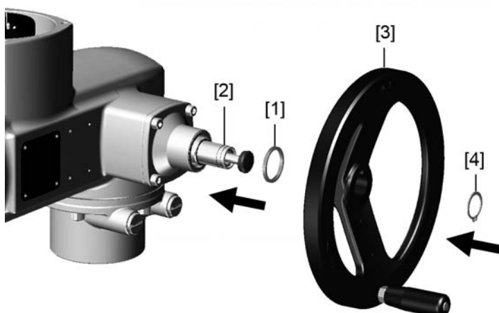
рис. 5: Маховик
