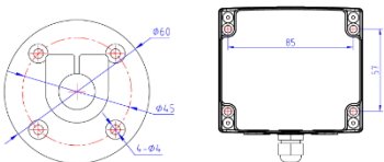
Установочные размеры, мм
