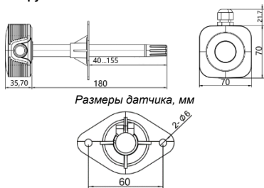
Установочные размеры, мм
