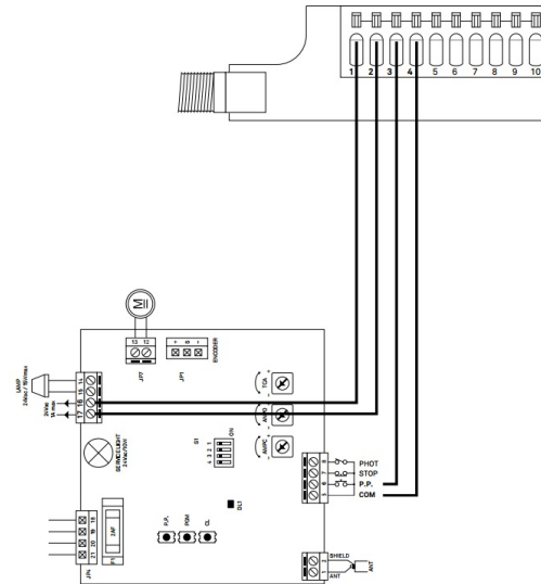
Рис. 2 Пример подключения одномодульного канала Proxi Gate к контроллеру ворот (управляющий элемент Beninca JM3)
