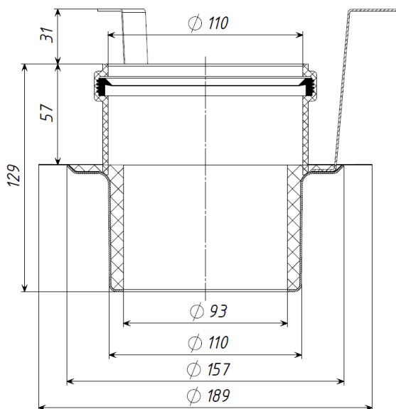
Рис. 1 – Размеры ТП-840
