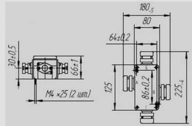
КП6 для вводов ВК25-В1,5-ЕхellU КП6П и КИ6П
