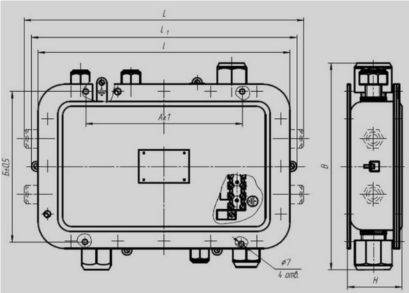
Рисунок3. Коробки с кабельными вводами (стальной)
