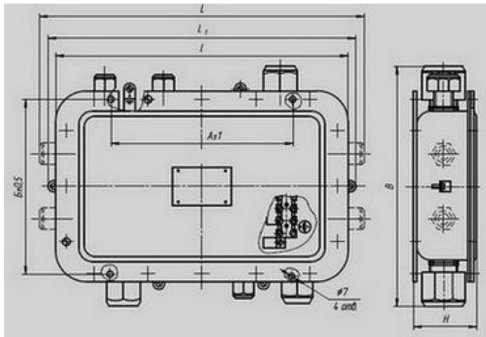
Рисунок1. Коробки с привертными сальниками (пластмассовый) Рисунок2 остальные см. рисунок1 Коробки с втулками пластмассовыми уплотнительными
