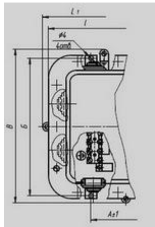
Рисунок1. Коробки с привертными сальниками (пластмассовый) Рисунок2 остальные см. рисунок1 Коробки с втулками пластмассовыми уплотнительными
