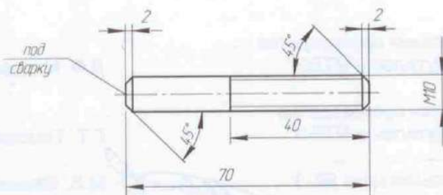
Деталь 2 Шпилька под приварку M10x70
