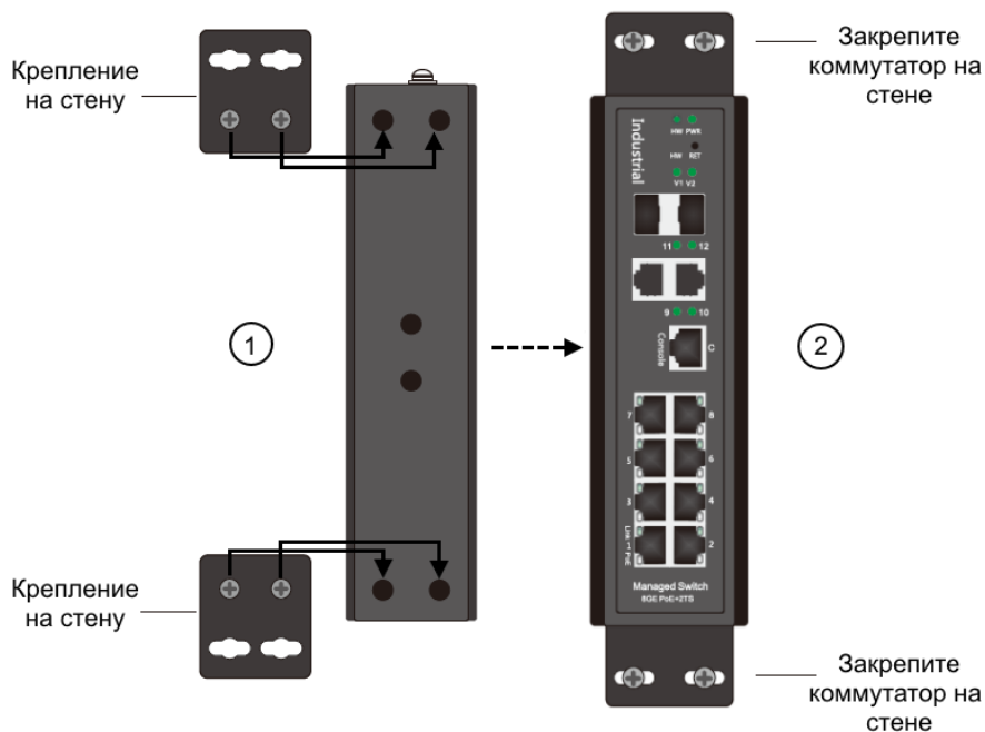
Рис. 13 Порядок монтажа коммутатора на стену
