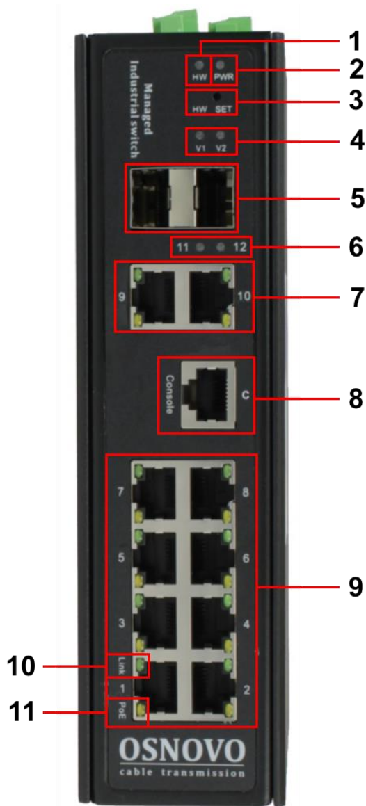
Рис.3 Коммутатор SW-80822/ILR, разъемы, кнопки и индикаторы на передней панели
