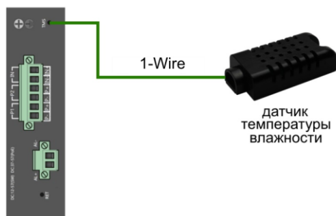
Рис.8 Схема подключения внешнего датчика температуры и влажности
