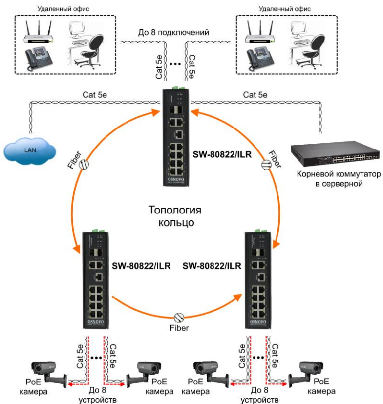
Рис. 7 Схема кольцевого подключения коммутатора SW-80822/ILR
