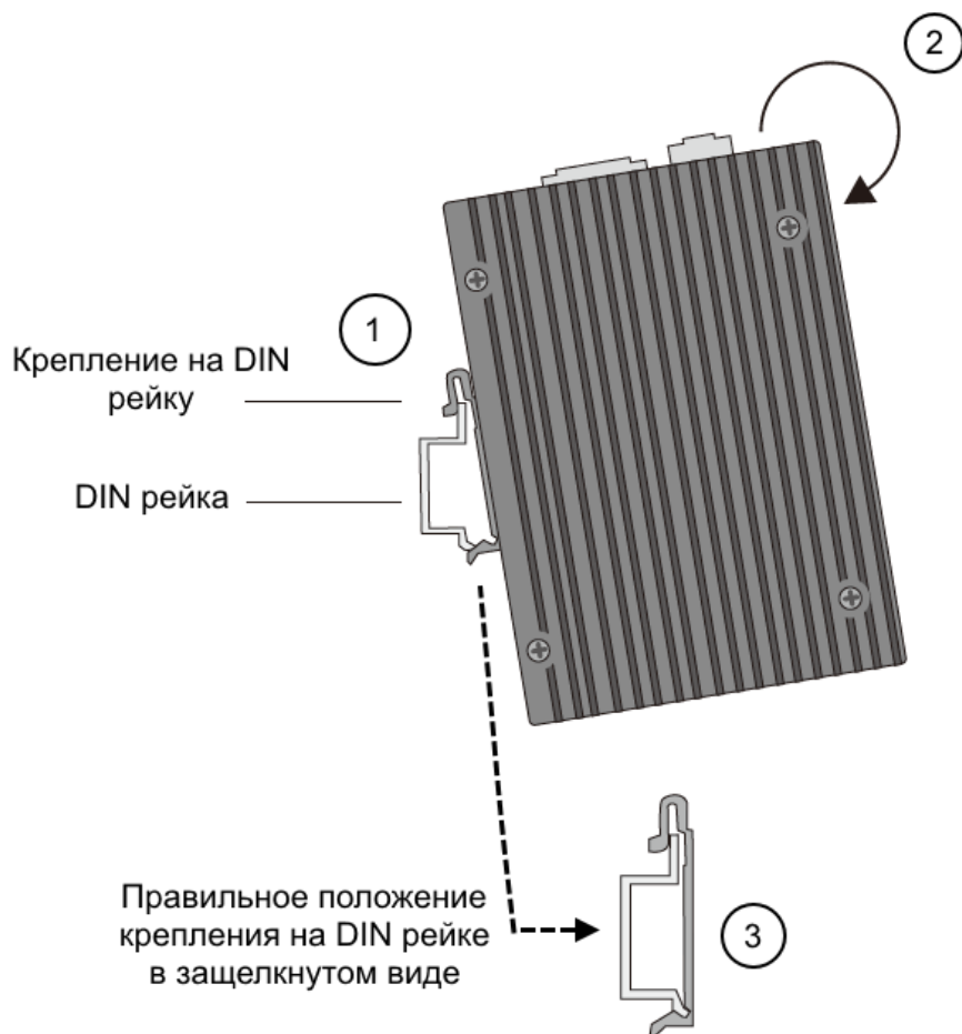
Рис. 12 Порядок монтажа коммутатора на DIN рейку
