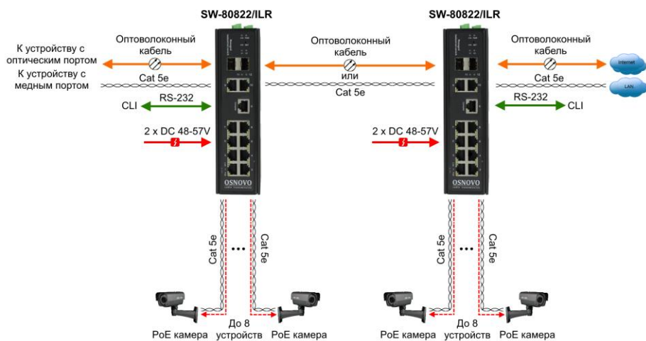
Рис. 6 Схема каскадного подключения коммутатора SW-80822/ILR
