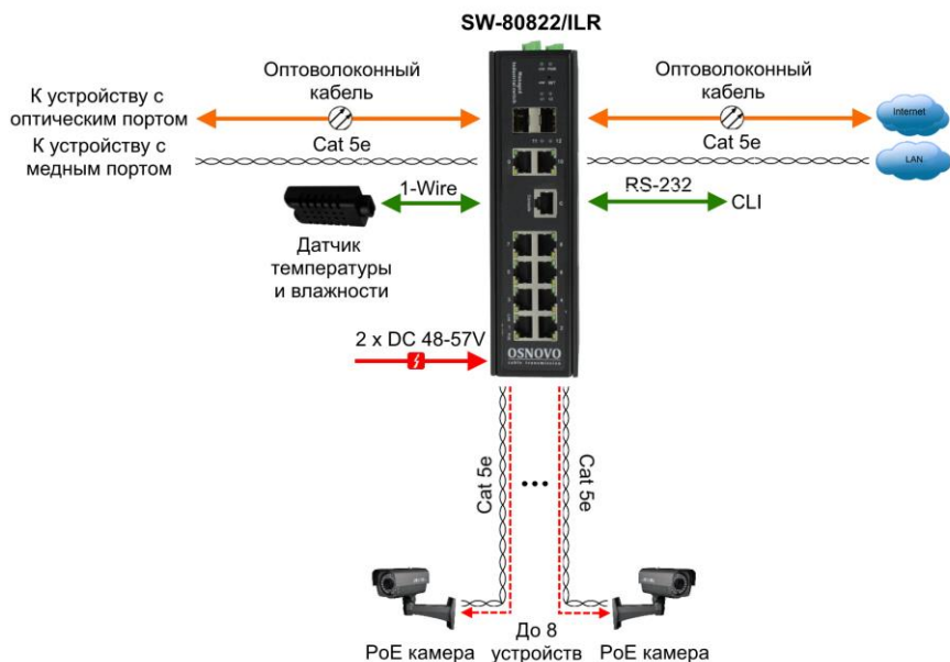
Рис. 5 Типовая схема подключения коммутатора SW-80822/ILR
