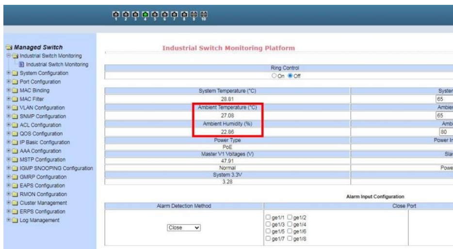
Рис.9 Контроль параметров температуры и влажности окружающей среды через Web-интерфейс коммутатора
