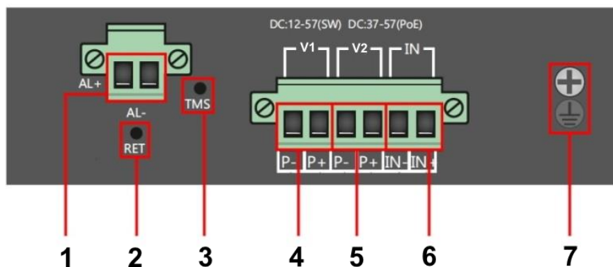
Рис.4 Коммутатор SW-80822/ILR, разъемы на верхней панели
