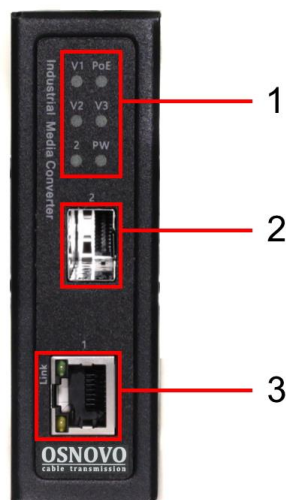
Рис.2 Медиаконвертеры ОМС-1000-11Х/І, ОМС-1000-11НХ/І, ОМС-1000-11ВХ-І разъемы, индикаторы, передняя панель.
