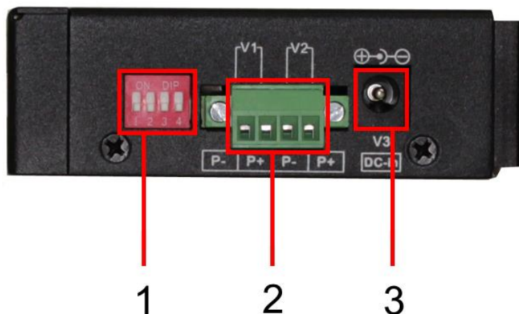
Рис.3 Медиаконвертеры ОМС-1000-11Х/І, ОМС-1000-11НХ/І, ОМС-1000-11ВХ-І, разъемы и переключатели, верхняя панель.
