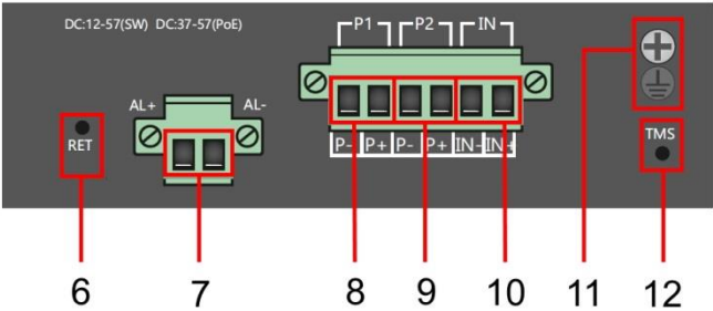
Рис. 4 Коммутатор SW-808010/ILS(port 90W 720W) разъемы и кнопки верхней панели
