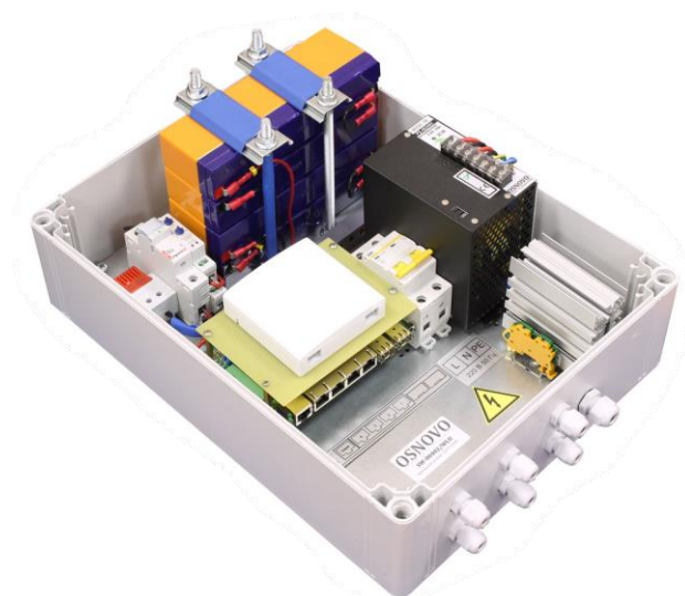
Рис. 2 Уличный коммутатор SW-80402/WLU, вид внутри
