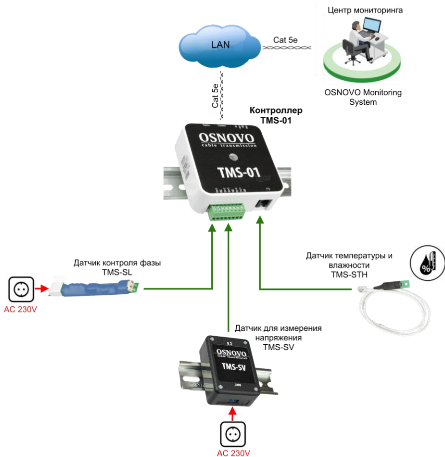
Рис.4 Типовая схема подключения контроллера TMS-01 с датчиками OSNOVO
