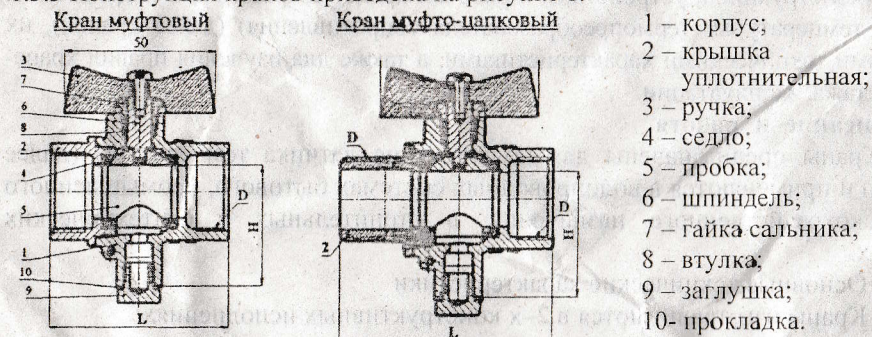
Рисунок 1. Краны шаровые для подключения датчика температуры.
