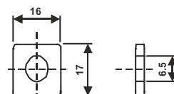
F4 (БОЛТ И ГАЙКА М6)
