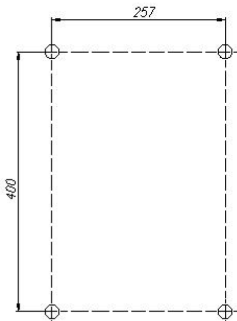
Рисунок 3 - Разметка сверления отверстий
