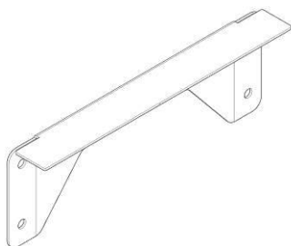
Накладка – 2 шт.
