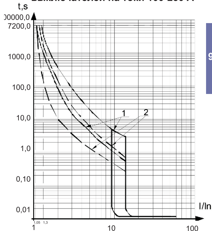
Время-токовые характеристики выключателей на токи 100-250 А
