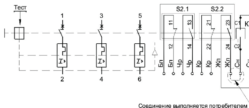
Схема электрическая принципиальная выключателя переменного тока трехполюсного исполнения с независимым расцепителем и вспомогательными контактами
