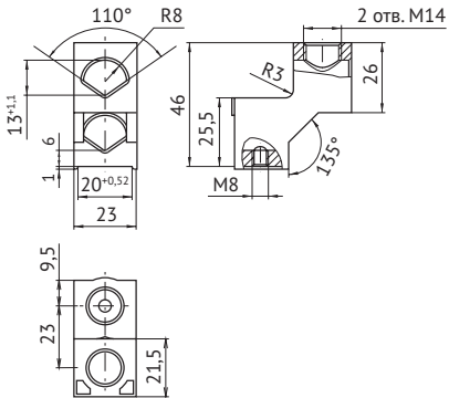
Зажим для присоединения двух кабелей сечением до 95 мм²
