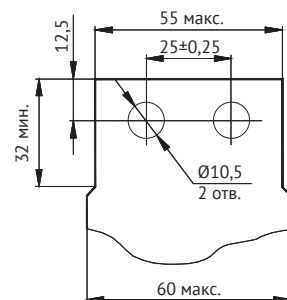
Форма и размер присоединяемой шины
