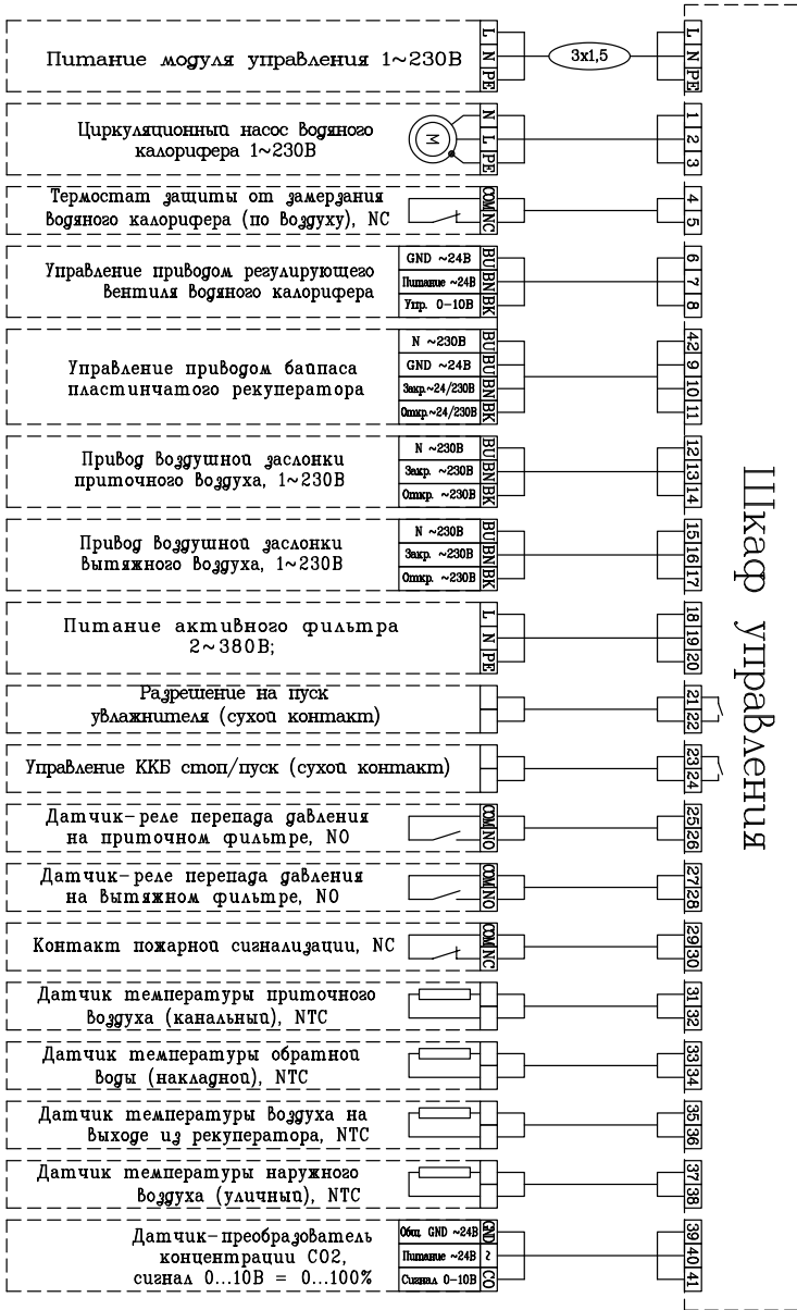
Схема ZPVP 1000 PW, ZPVP 1500 PW
