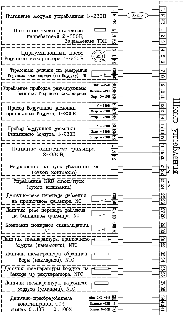
Схема ZPVP 450 PW, ZPVP 800 PW
