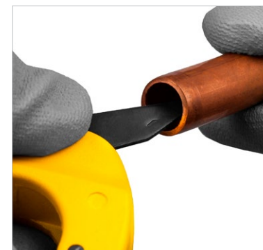
Нож для снятия фаски
