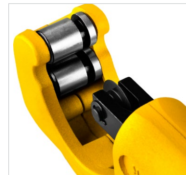
Ролики для фиксации развальцованных труб
