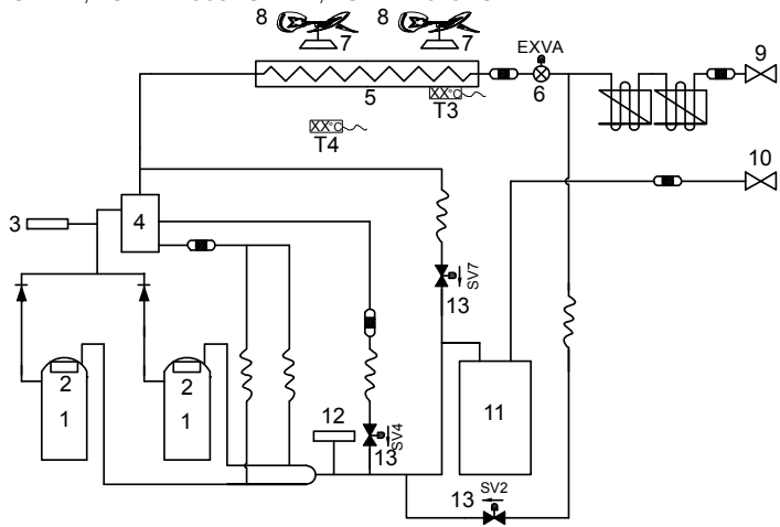
Описание компонентов гидравлической схемы
