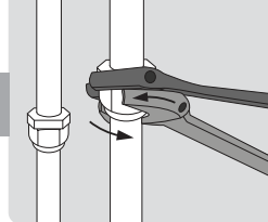
Соединение труб хладагента
