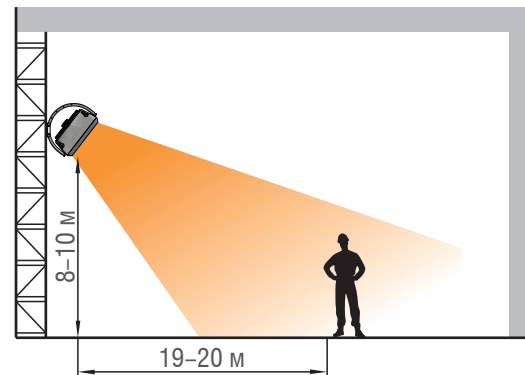
Настенный монтаж
