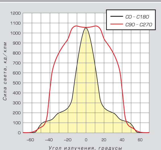
Диаграмма направленности СТАЙЛ СМ
