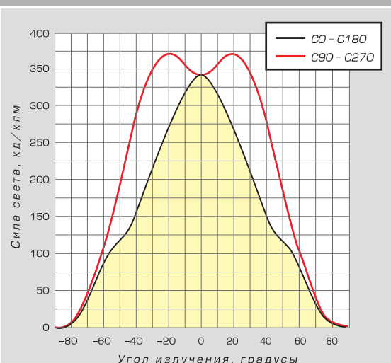
Диаграмма направленности ЭВОЛЮШН СМ
