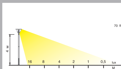
Диаграмма освещенности для MAR-B-T-DF2
