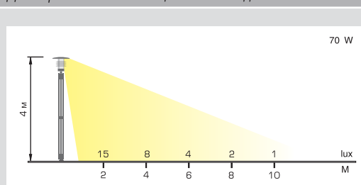
Диаграмма освещенности для AKS-70N
