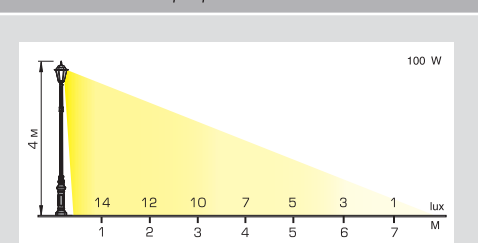
Диаграмма освещенности для светильника «Петергоф» с прозрачным стеклом
