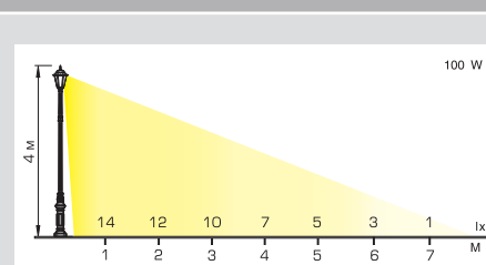
Диаграмма освещенности для светильника «Павловск» с прозрачным стеклом
