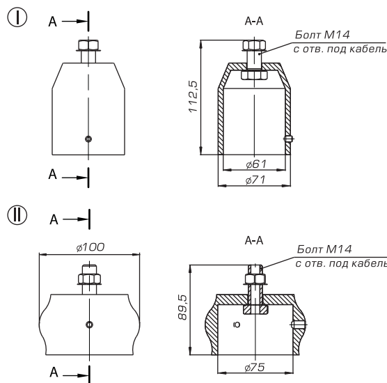
Установочные (монтажные) комплекты (МК) для нижнего крепления (D)
