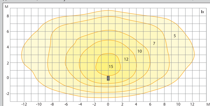
для ST 50, высота установки – 8 м
