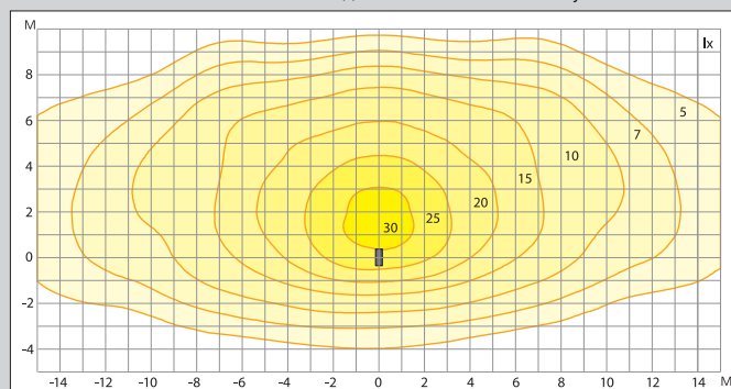
для ST 100, высота установки – 8 м
