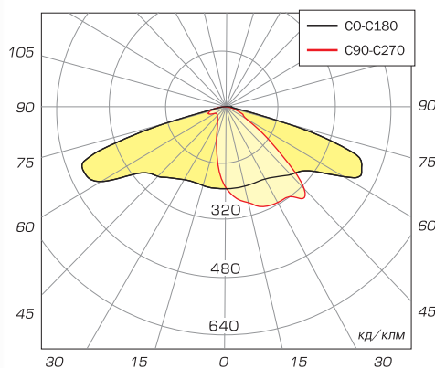
Диаграмма направленности, cd/Klm
