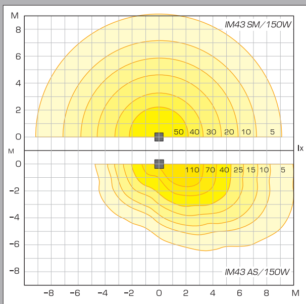
Диаграмма освещенности для IM43/150W Площадка 20 x 20 метров
