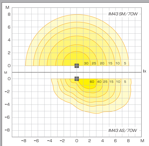
Диаграмма освещенности для IM43/70W Площадка 20 x 20 метров
