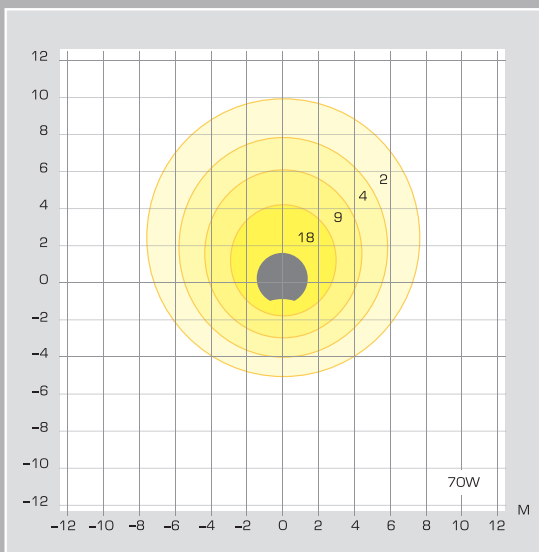
Диаграммы освещенности, lx
