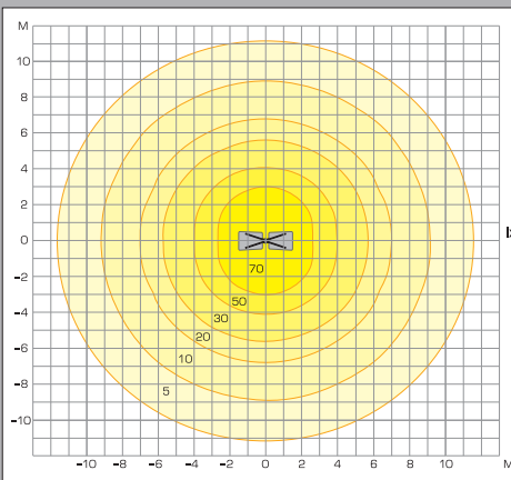
для SAY60/2, lx
