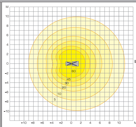
для SAY60/3, lx
