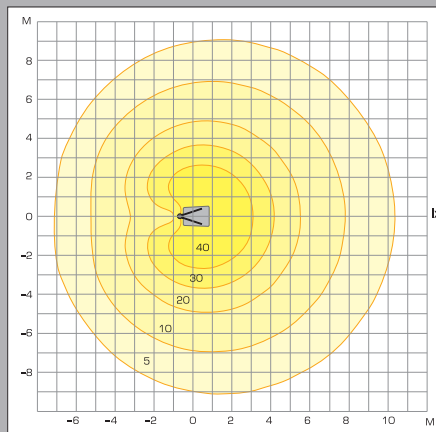
Диаграммы освещенности
