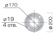
вариант 1 фланцевое соединение
