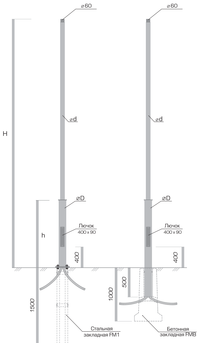
вариант 1 фланцевое соединение
